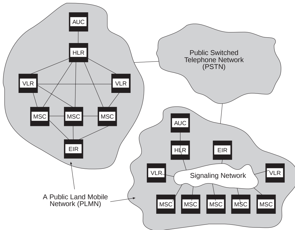
Fig. 5.1 GSM PLMN
